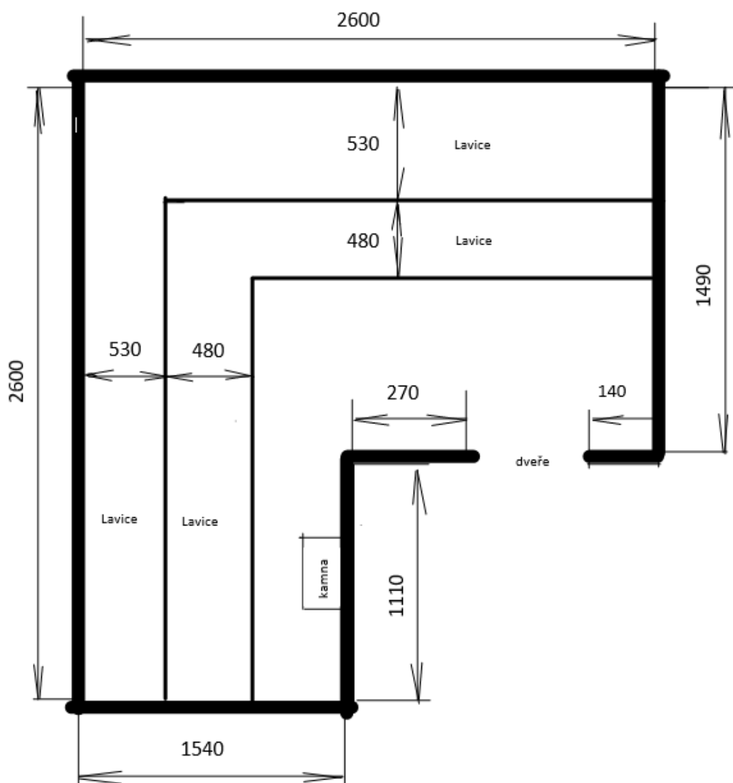
Obr. Rozměry sauny (v mm)
